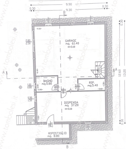
Villa Valtella Planimetria
