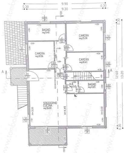
Villa Valtella Planimetria
