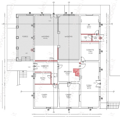
PIANO TERRA RIALZATO
